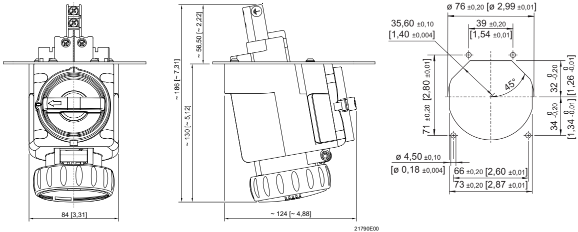
8570/25-3.. SolConeX flange socket
