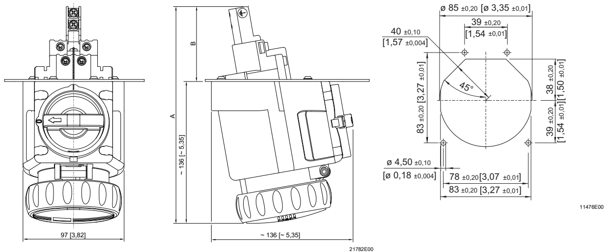
8570/25-4.. et 8570/25-5.. Prise de courant à bride SolConeX
