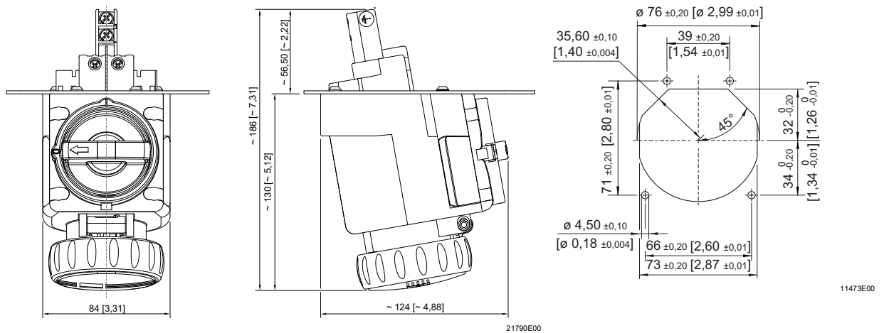
8570/25-3.. Prise de courant à bride SolConeX
