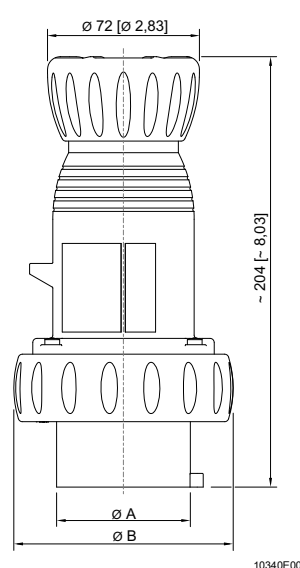
8571/12 SolConeX 插头
