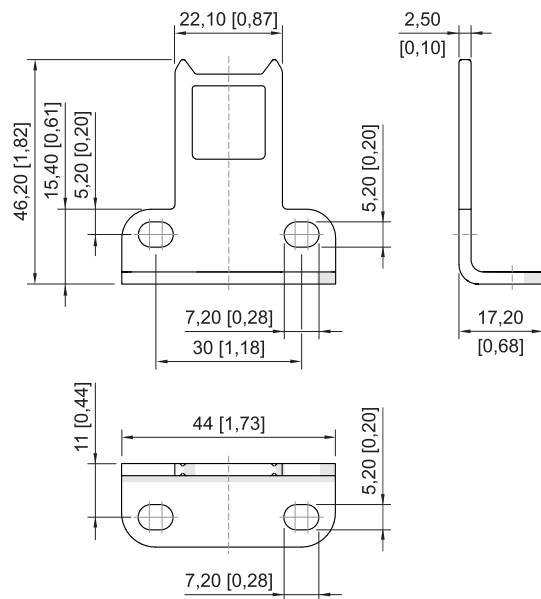
Угловой приводной механизм для предохранительного выключателя
