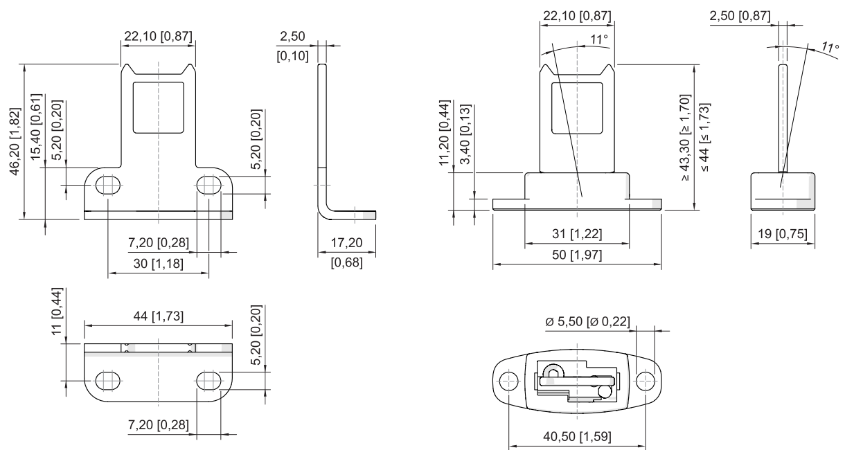
Betätiger für Sicherheitsschalter gerade
