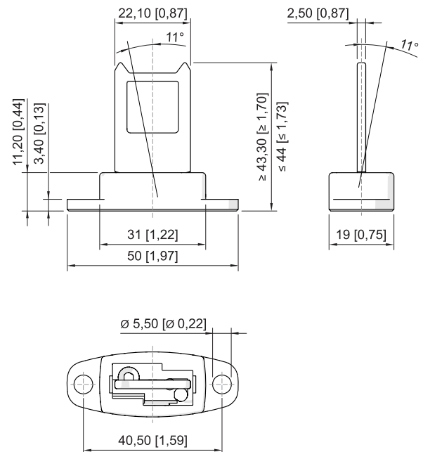
Прямой приводной механизм для предохранительного выключателя
