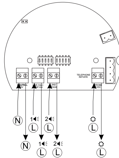
Schéma électrique pour tensions alternatives
