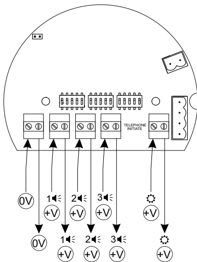
Schéma électrique pour tensions continues
