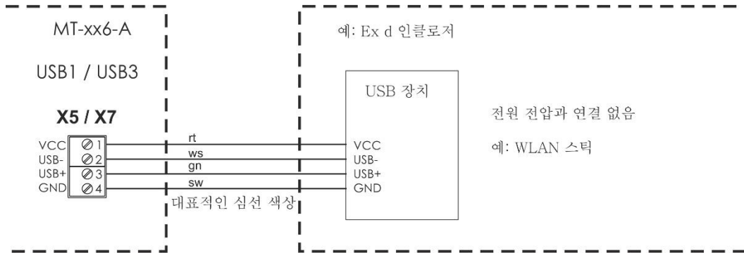
결선도 유형 1(예: WLAN 스틱)
