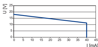
Ausgangskennlinie 9475/32-04-12
