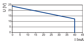
Ausgangskennlinie 9475/32-04-22
