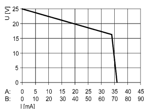
Ausgangskennlinie 9175/0-16-11; 9176/0-16-00
