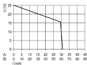
Ausgangskennlinie 9176/0-15-00
