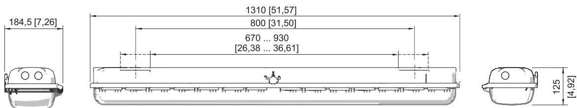
Baugröße 4
