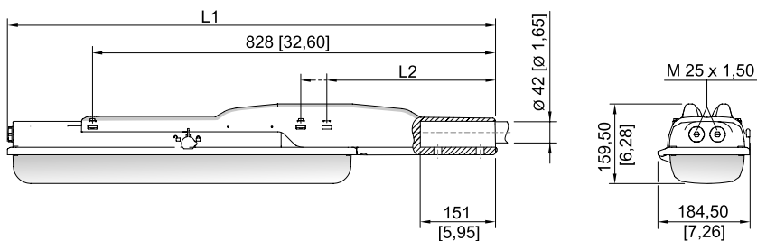
Baugröße 6
