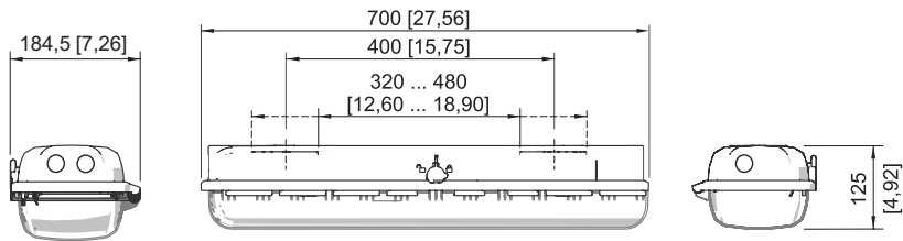
Baugröße 2
