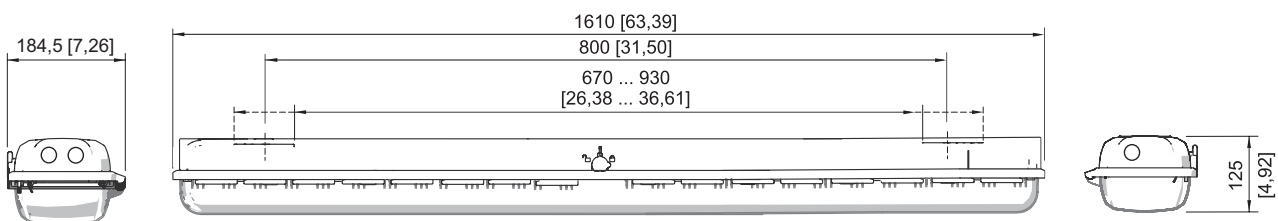
Baugröße 6
