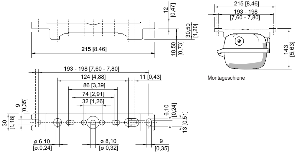
Montageschiene
