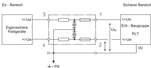
Zwei-Kanal-Sicherheitsbarrieren Potential: ~ / ~
