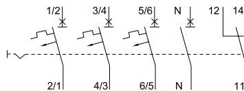
3-polig+N, Hilfskontakt 1 Wechsler
