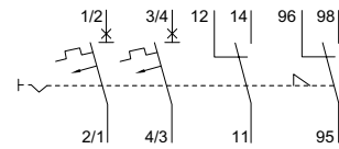
2-polig, Hilfskontakt 1 W + Fehlersignalkontakt 1 W
