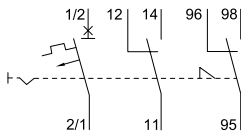
1-polig, Hilfskontakt 1 Wechsler + Fehlersignalkontakt 1 Wechsler
