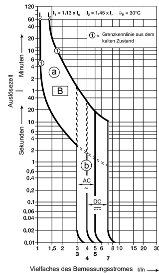
Auslösecharakteristik B
