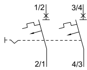
2-polig, ohne Hilfskontakt
