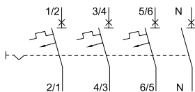
3-polig+N, ohne Hilfskontakt
