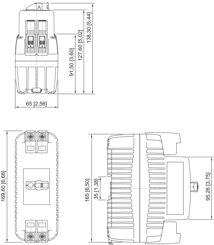
8530/1; 2 Teilungseinheiten
