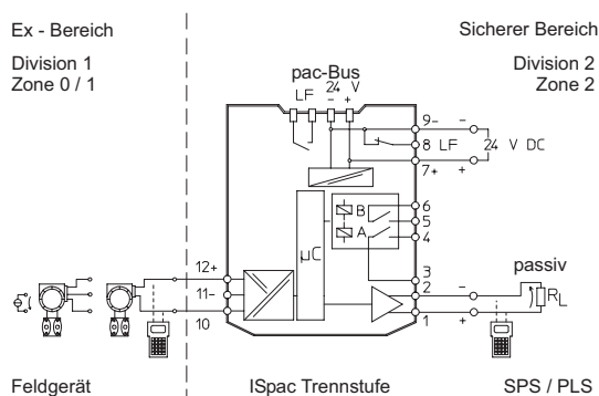
Anschlussplan 9162/13-11-14
