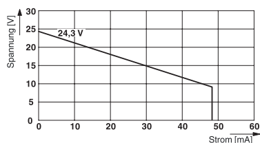
Ausgangskennlinie 9275/10-24-48-11
