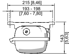
Montageschiene
