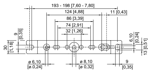
Montageschiene
