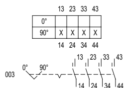
Schaltabwicklung 8006/4-003-00
