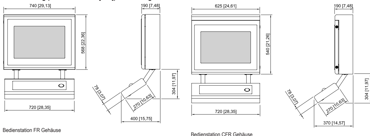
Bedienstation CFR Gehäuse
