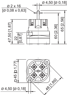
8008/2-0 Steuerschalter 1- oder 2-polig
