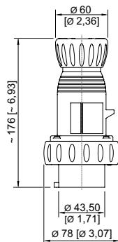
Stecker 3-polig
