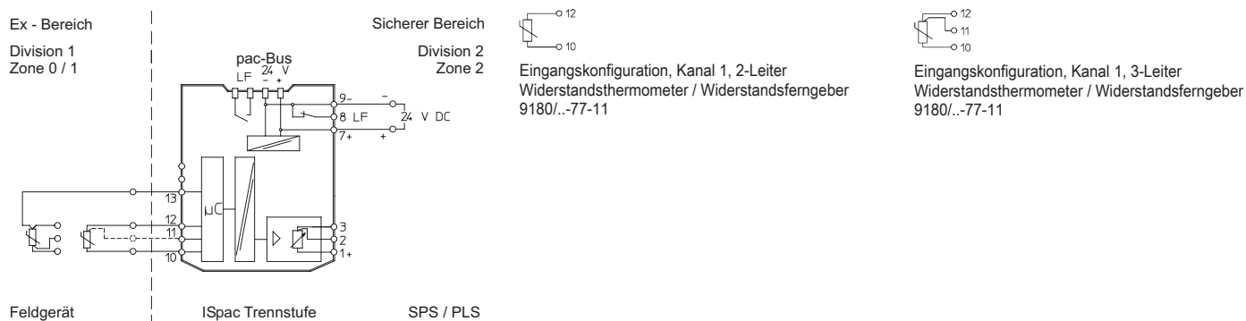
Anschlussplan 9180/1.-77-11
