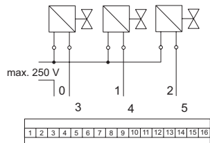
Anschlussplan 9477/12-08-12
