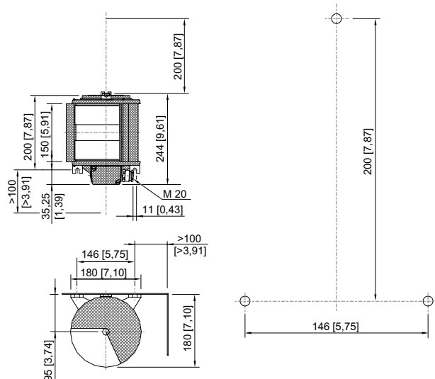
TEF 2850 Sektorlaterne
