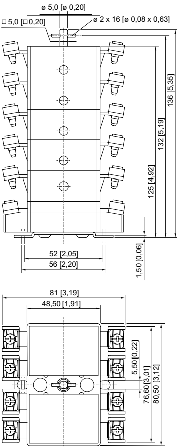
Last- und Motorschalter Reihe 8006/4, 9-polig und 10-polig
