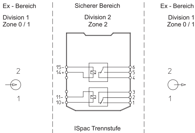
Anschlussplan 9172/22-11-00
