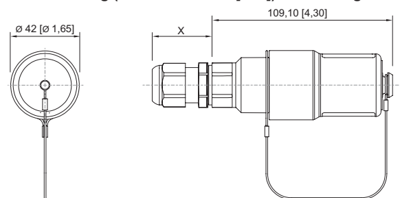
8595/1 Kupplung X = abhängig von der verwendeten Kabelverschraubung
