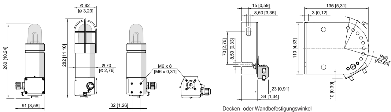
Blitzleuchte 6161
