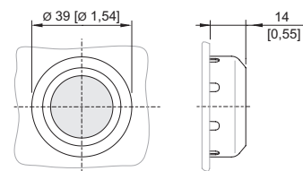
8602/3-001 Drucktaster Betätigungsverstärker mit axialer Betätigung
