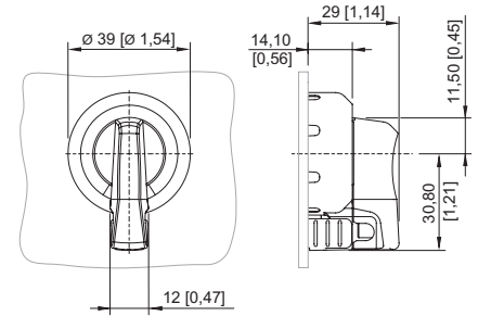
8602/3-734 Drehgriff, 1-fach abschließbar Betätigungsvorsatz mit radialer Betätigung
