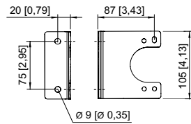
L-förmiger Winkel
