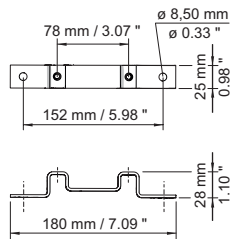
Befestigungsbügel
