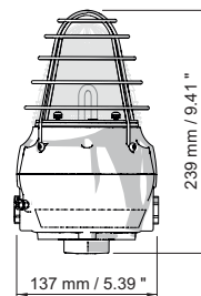
FX15 Blitzleuchte
