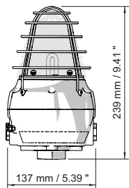
FX15 Blitzleuchte
