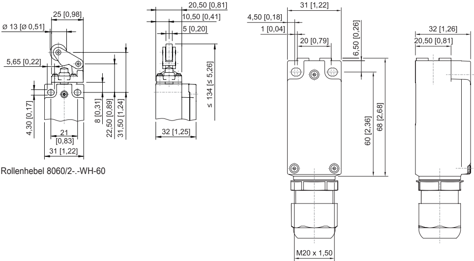
Schleichschaltglied 2 Öffner 8060/-3; 807-/2-3
