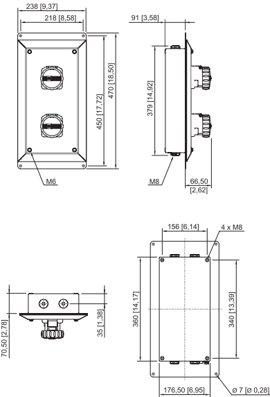
8150/5-V88 mit 8572/15, 16 A
