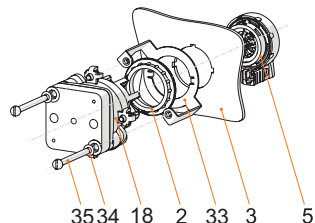
Montage Fronteinbau mit Steuerschalter Reihe 8008
