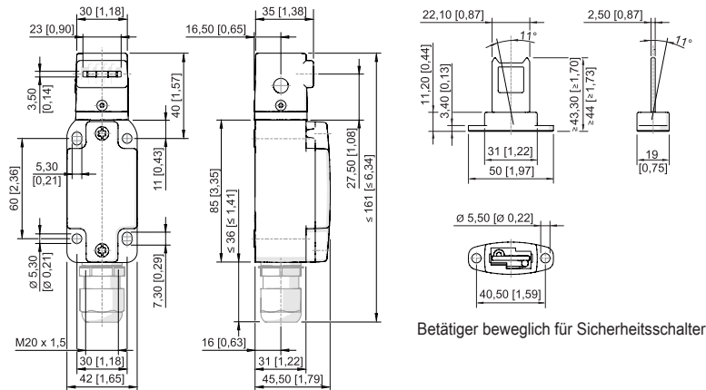
Sicherheitsschalter 8070/2.-AZ-U50
