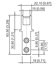
Sicherheitsschalter 8070/2.-AZ-U50
