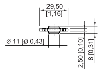
Betätiger für Sicherheitsschalter gerade
