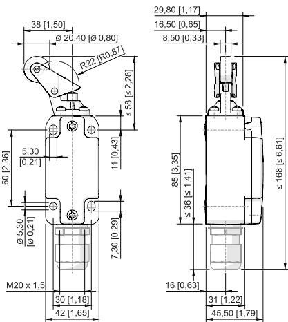
Rollenhebel 8070/2-2-WPH-U60
