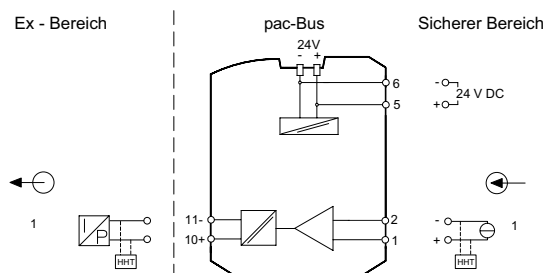
Anschlussplan 9265/16
