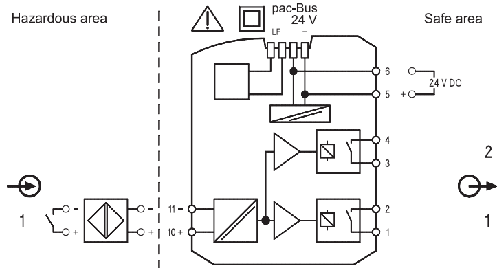
Anschlussbild 9270/11-17-15
