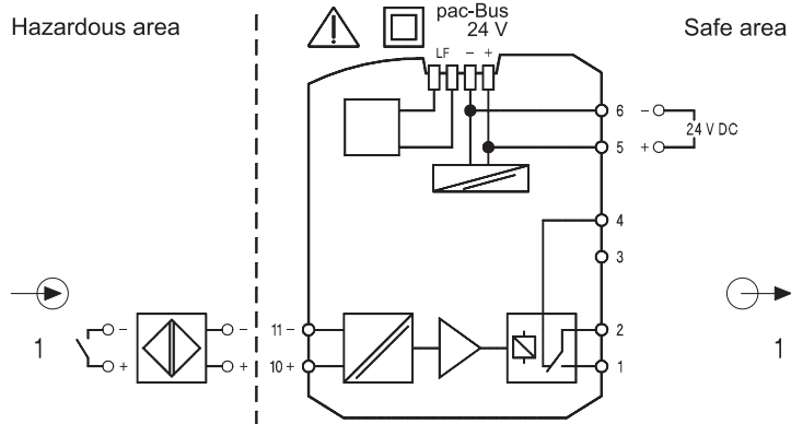
Anschlussbild 9270/11-16-14
