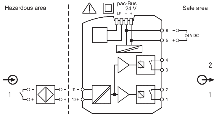
Anschlussbild 9270/11-17-15
