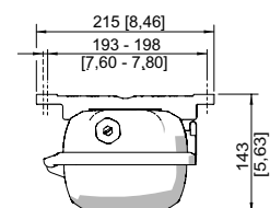
Montageschiene
