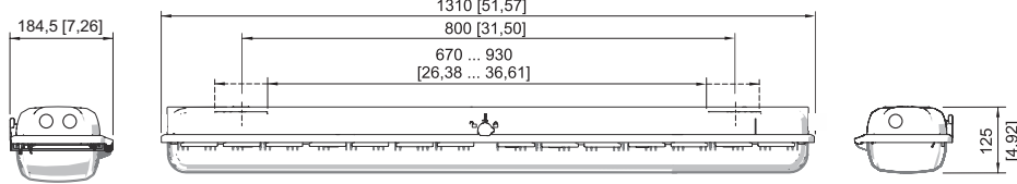
Baugröße 4
