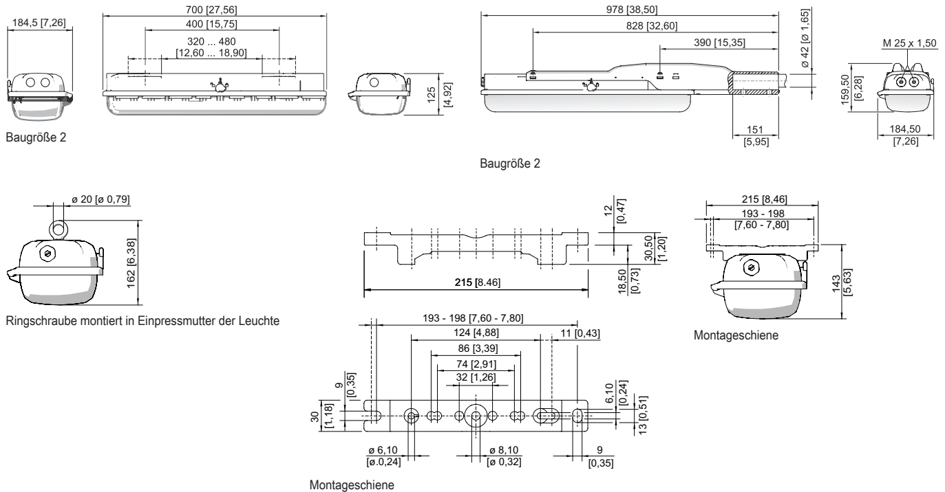
Montageschiene
