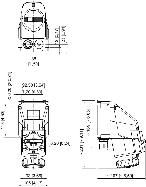
Wandsteckdose 3-polig
