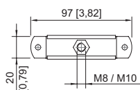
Montageklammer Gewinde
