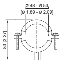
Montageklammer Gewinde
