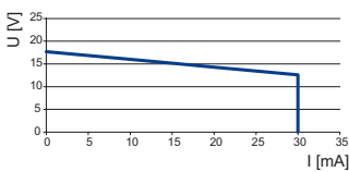
输出特性曲线 9475/32-08-52, 9475/33-08-50
