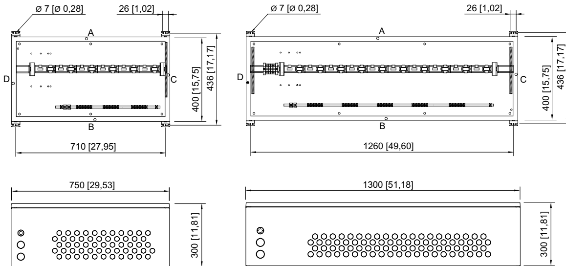
1 x 6 插槽总线导轨 订货号 282643
