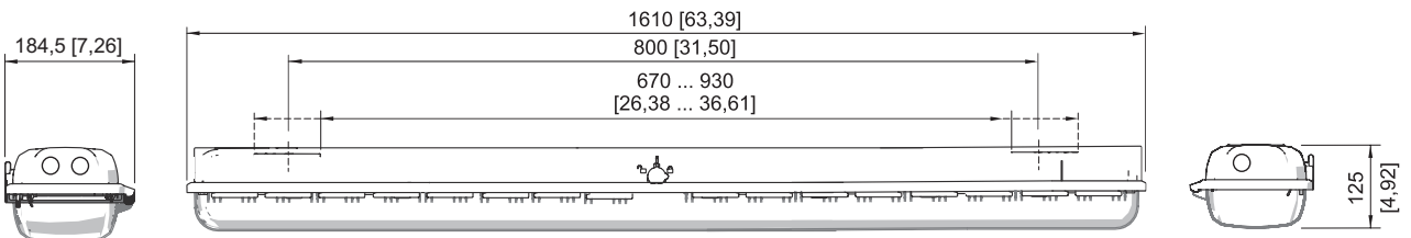
设计尺寸 6
