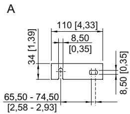
壁装支架装配在安装导轨中
