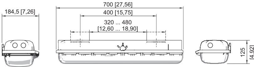
设计尺寸 2
