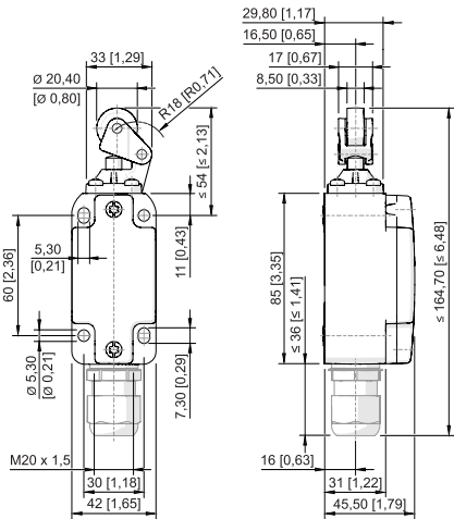
Roller lever 8070/2--WH-U60
