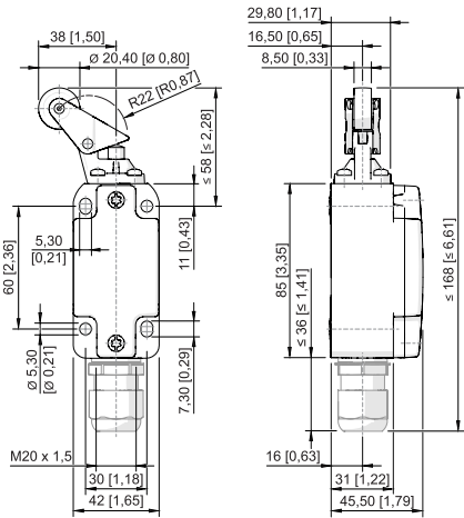
Roller lever 8070/2-3-WPH-U60
