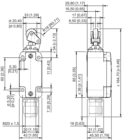
Roller lever 8070/2-4-WH-U60
